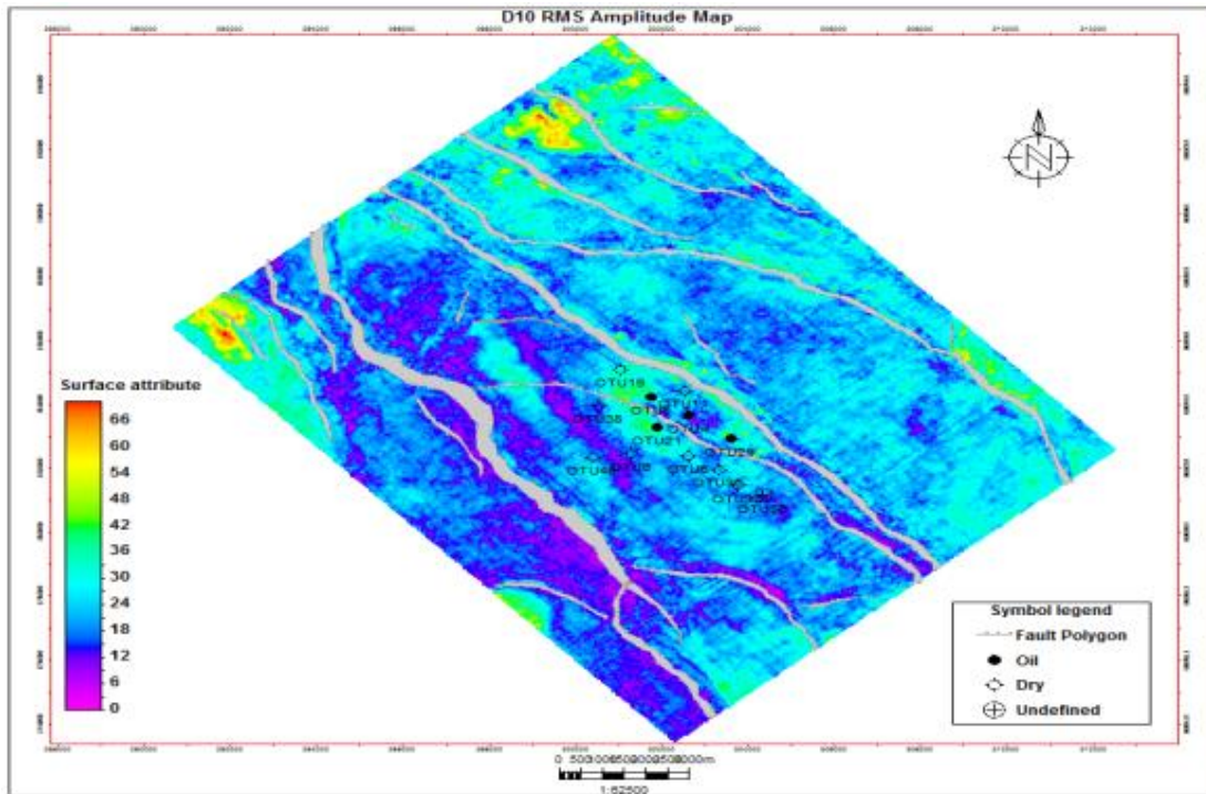
Fig. 15. RMS amplitude for horizon D10
